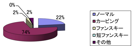
スキー用具
