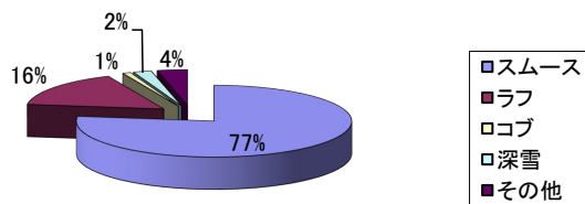
雪面状況
